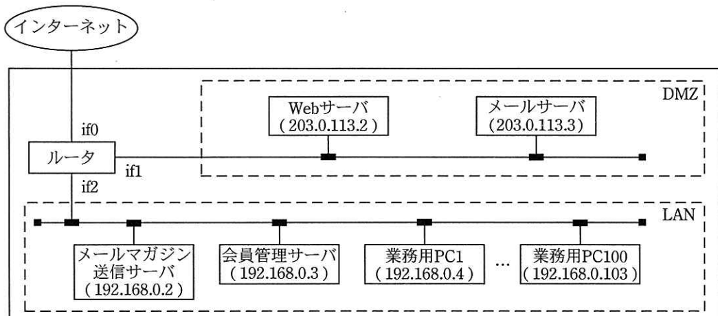
図1 A社のネットワーク構成
